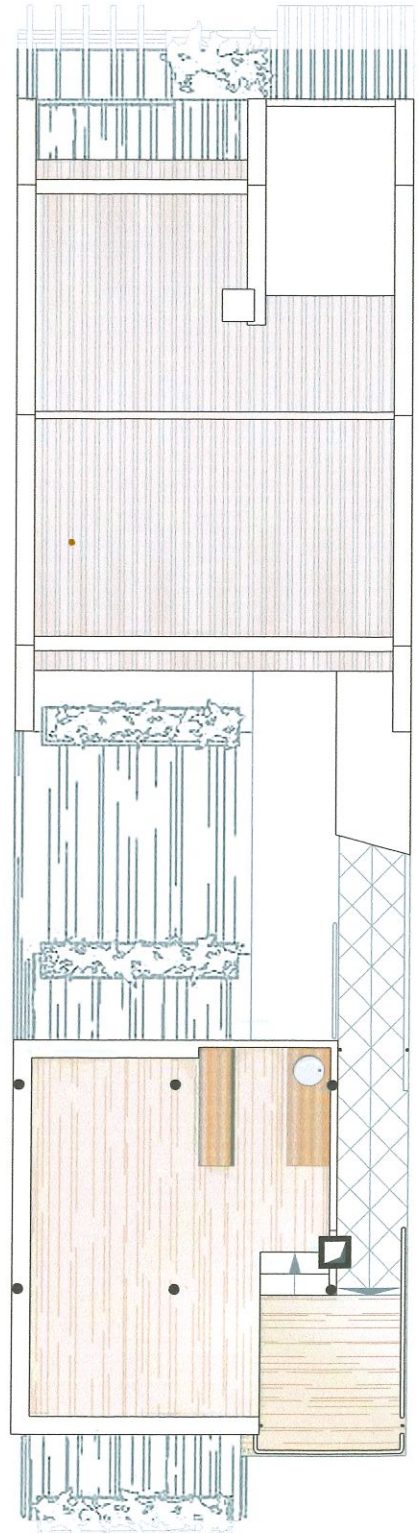
Cobertura Roof
