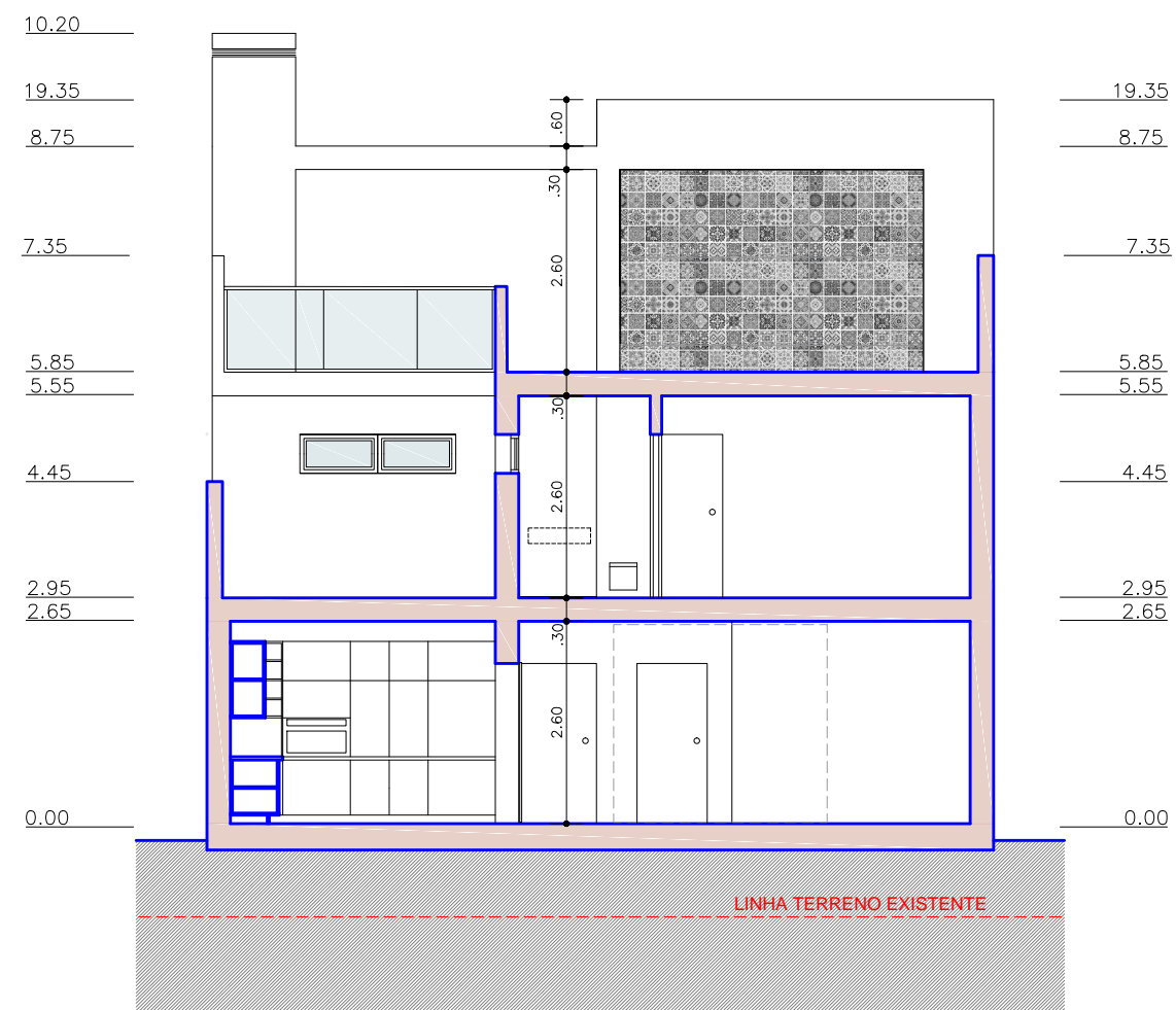
CORTE B-B
