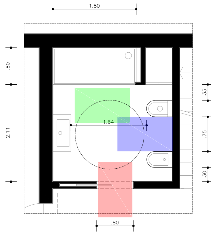
PORMENOR I.S. ACESSIVEIS - ESC. 1/50
