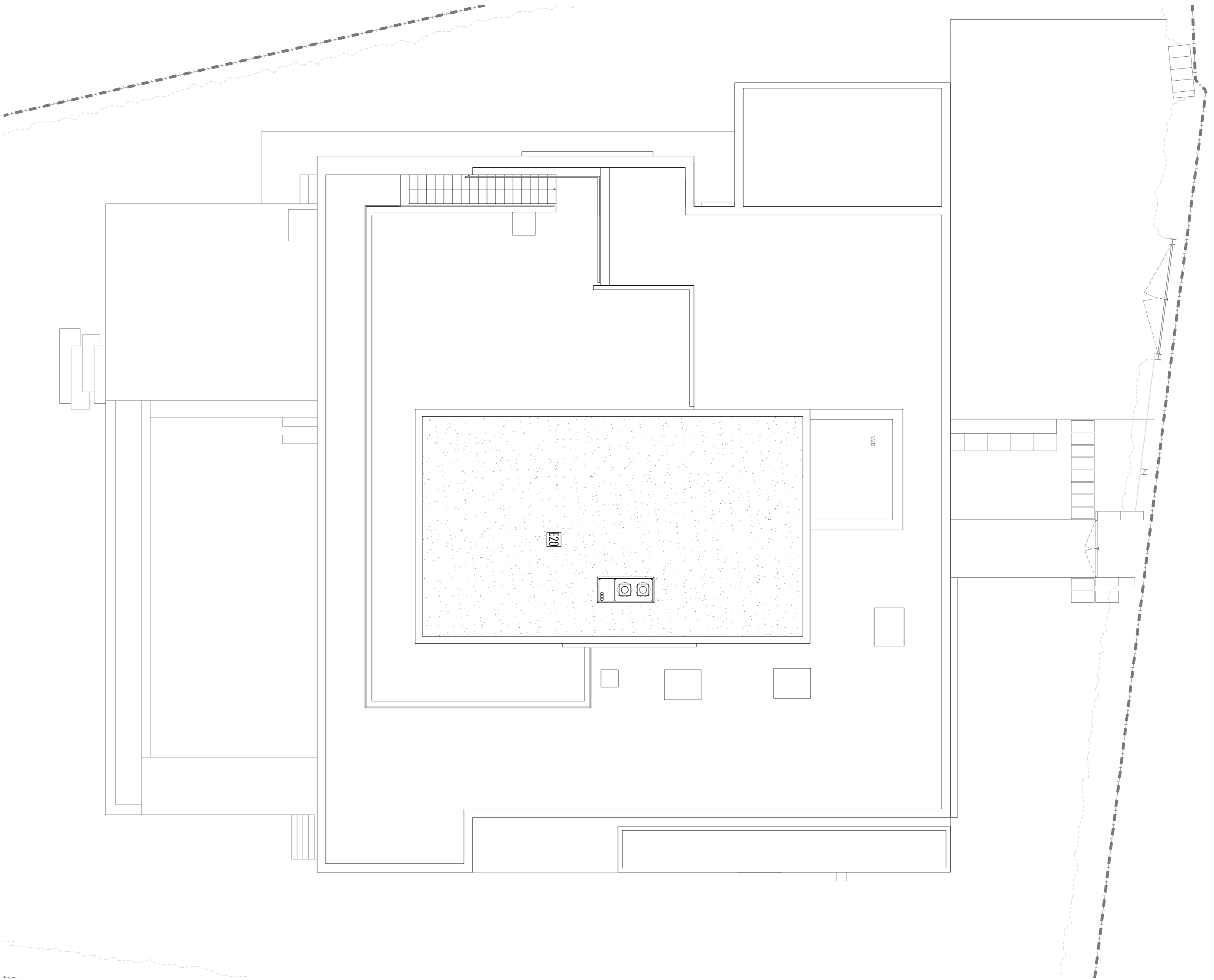
Pianta DA COPERTURA
