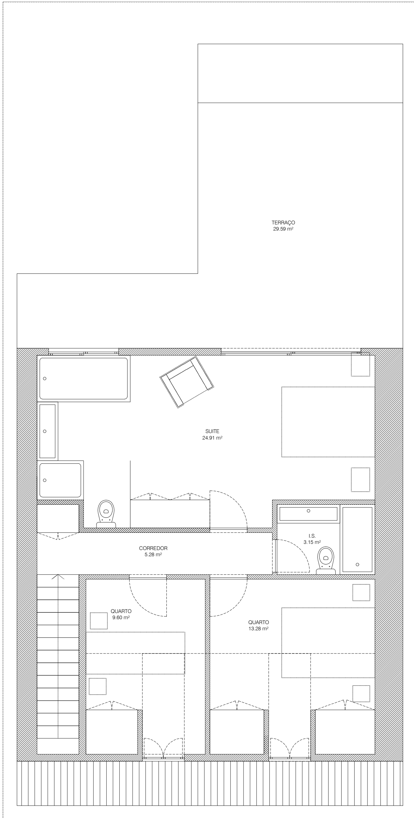
PLANTA PISO 2
