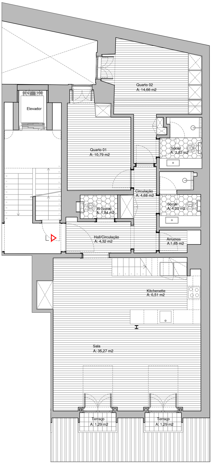
APARTAMENTO L PISO 5 escala 1:100
