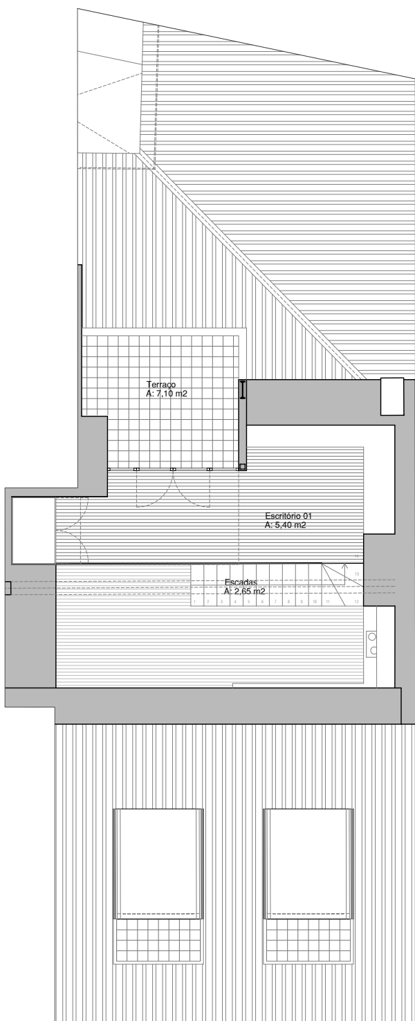
APARTAMENTO L MEZZANINE escala 1:100
