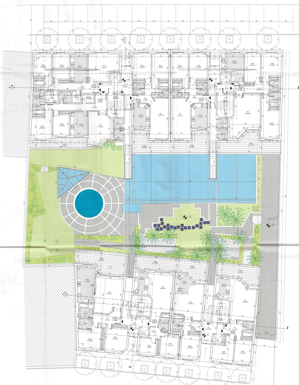
Planta do Rés-do-chão 1:100
