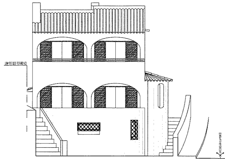
alçado A4/SUDESTE
