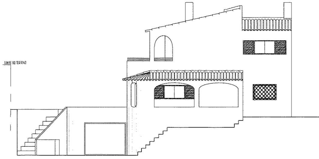
alçado A1/SUESTE
