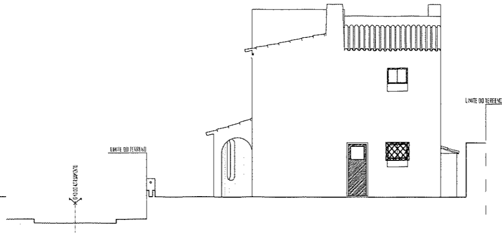
alçado A2/NORDESTE
