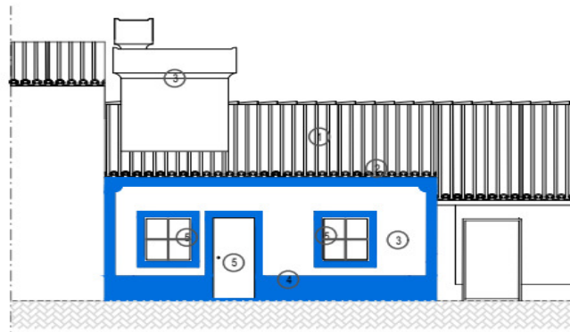
Alçado Principal Proposto
