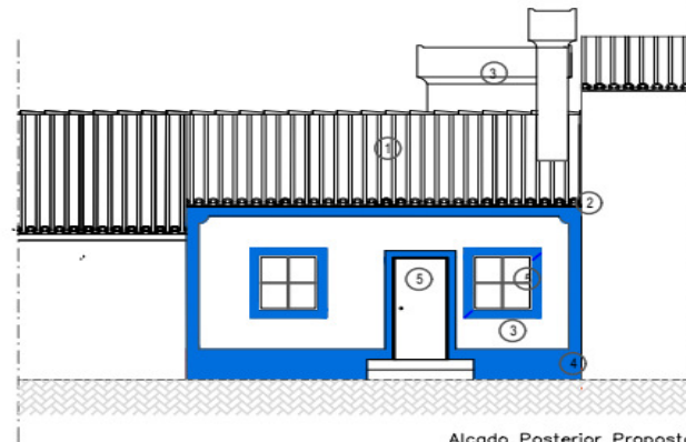
Alçado Posterior Proposto
