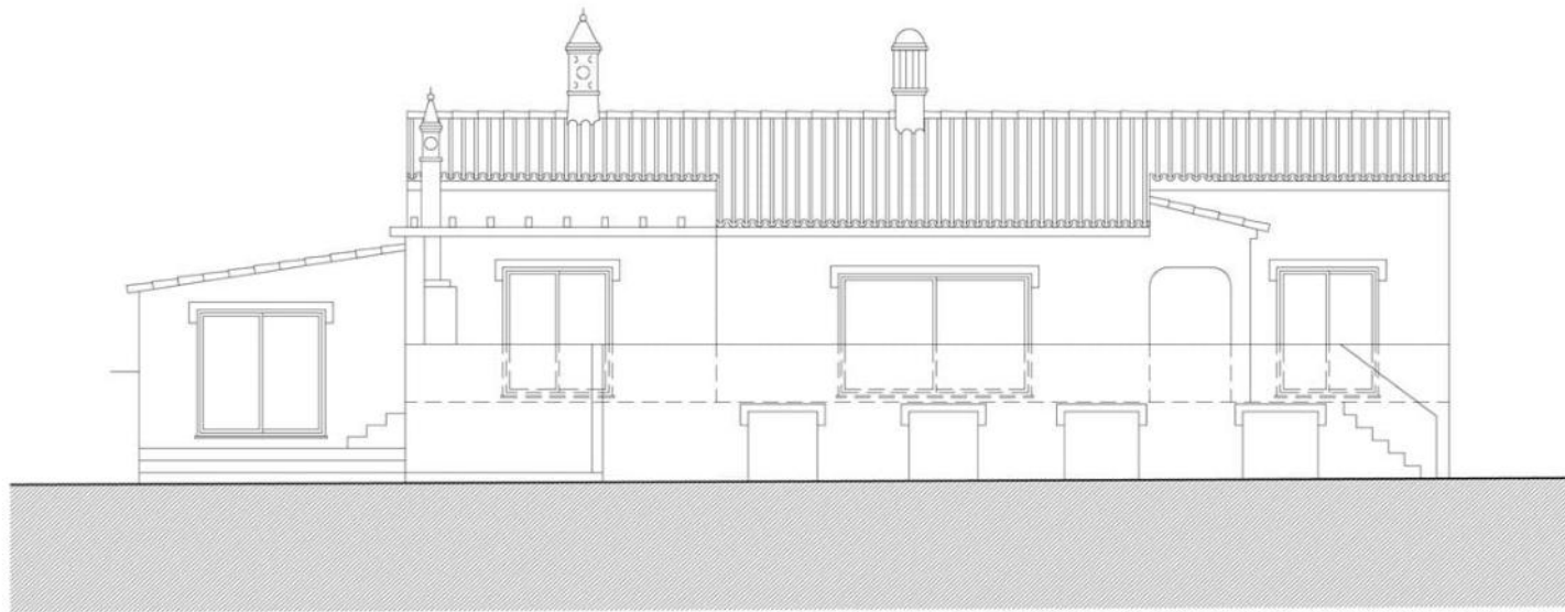
ALÇADO PRIINCIPAL
