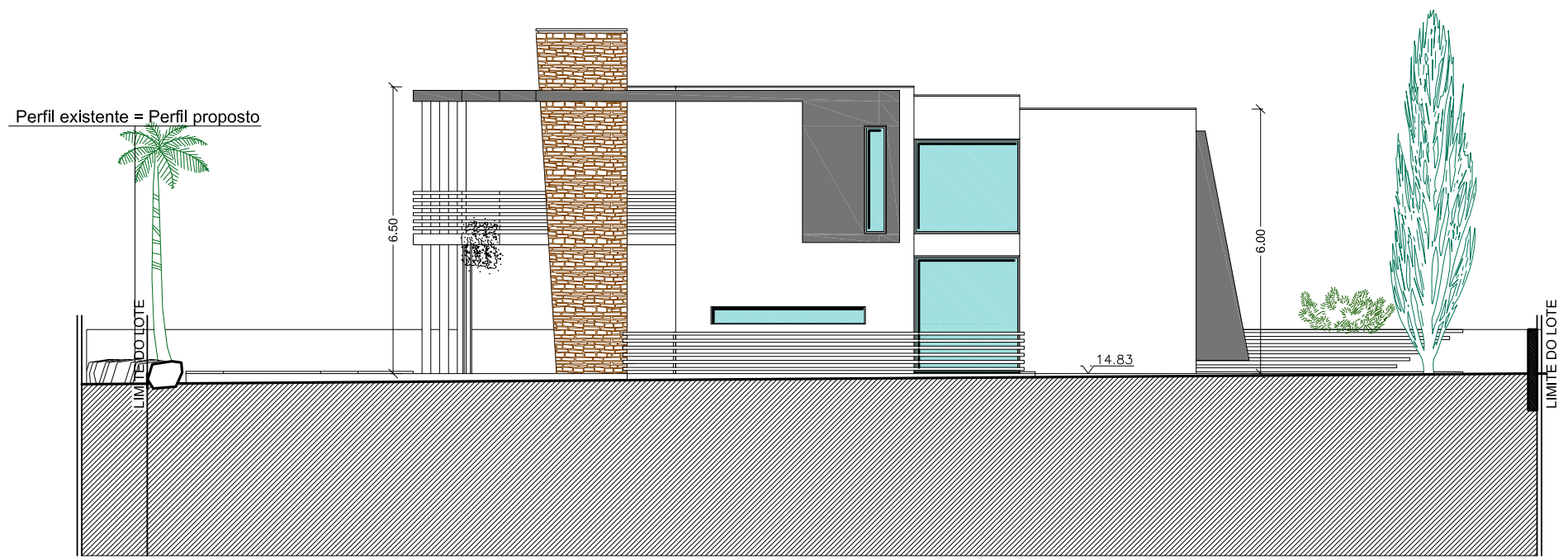
ALÇADO SUL
