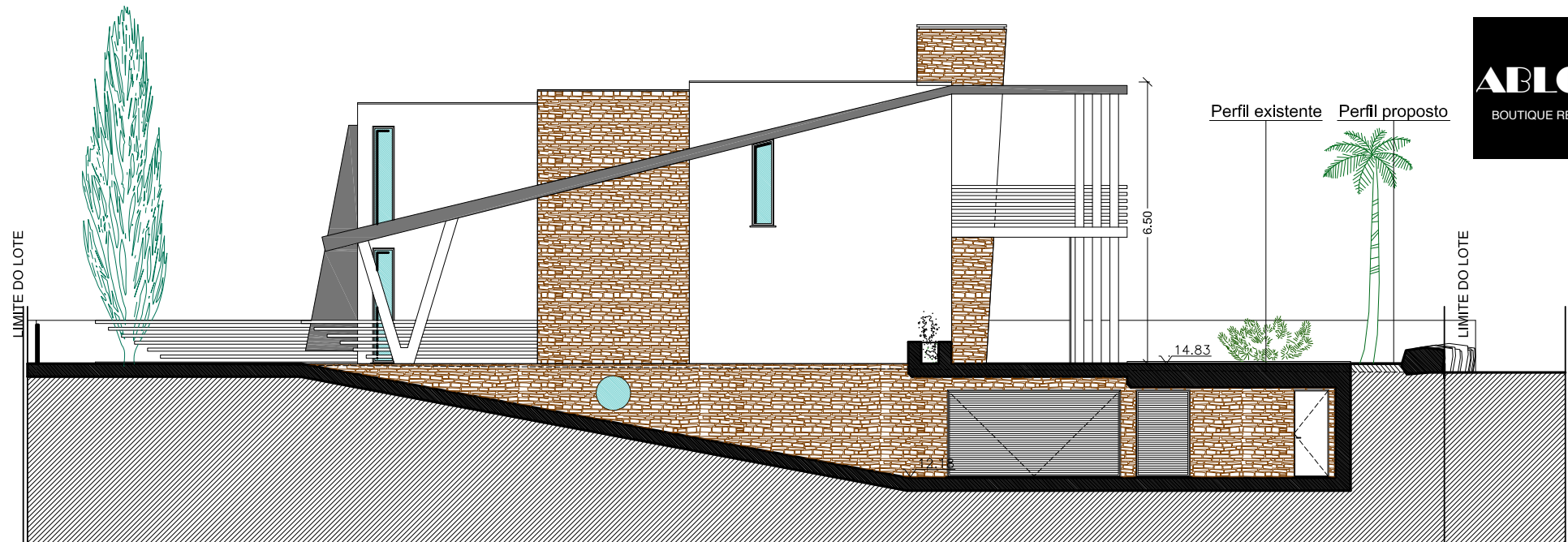
ALÇADO NORTE
