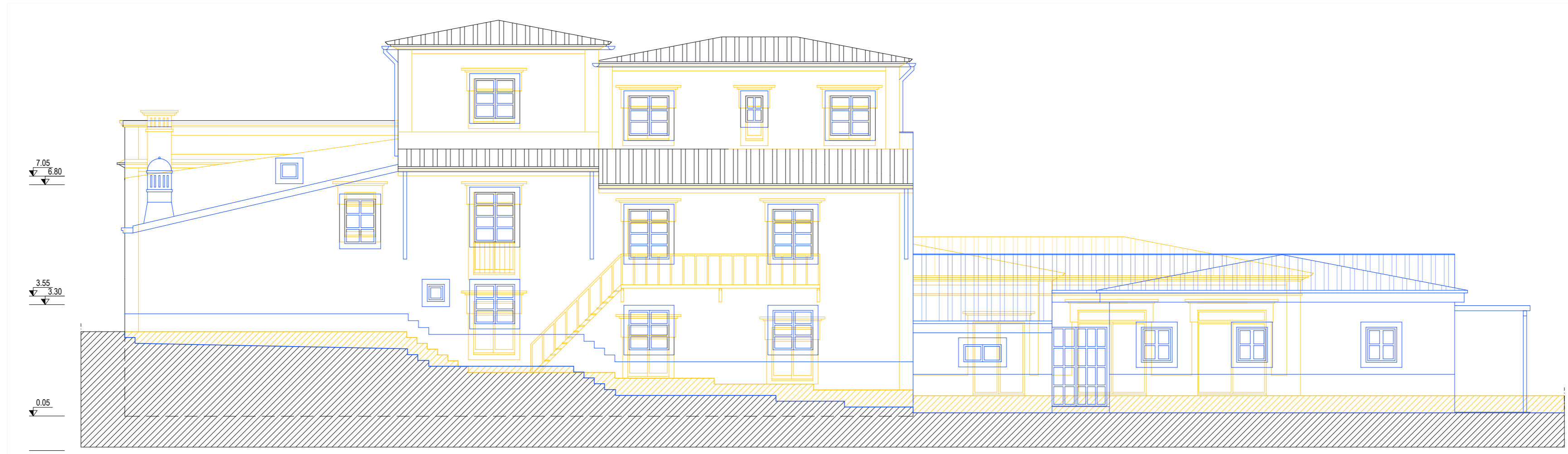
ALÇADO POENTE
