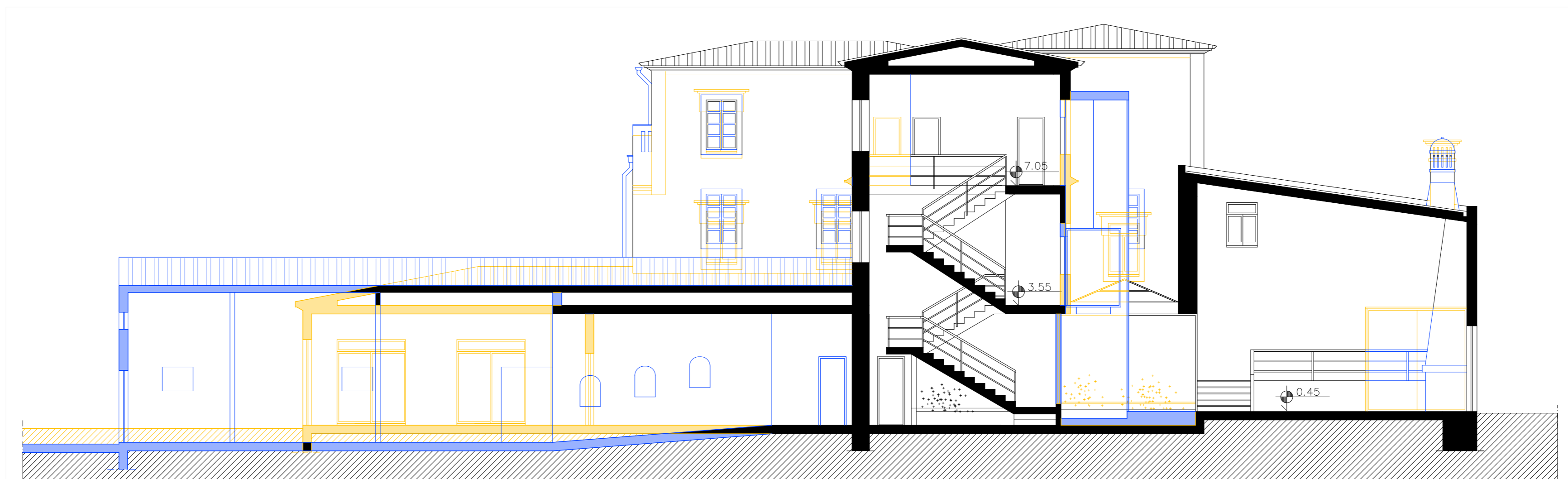
CORTE B
