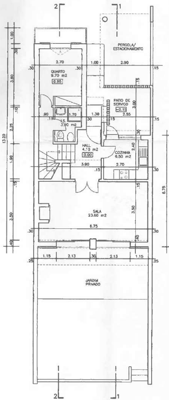
PLANTA PISO 0
