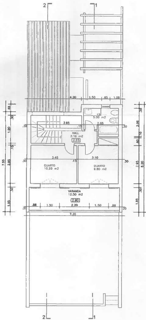
PLANTA PISO 1
