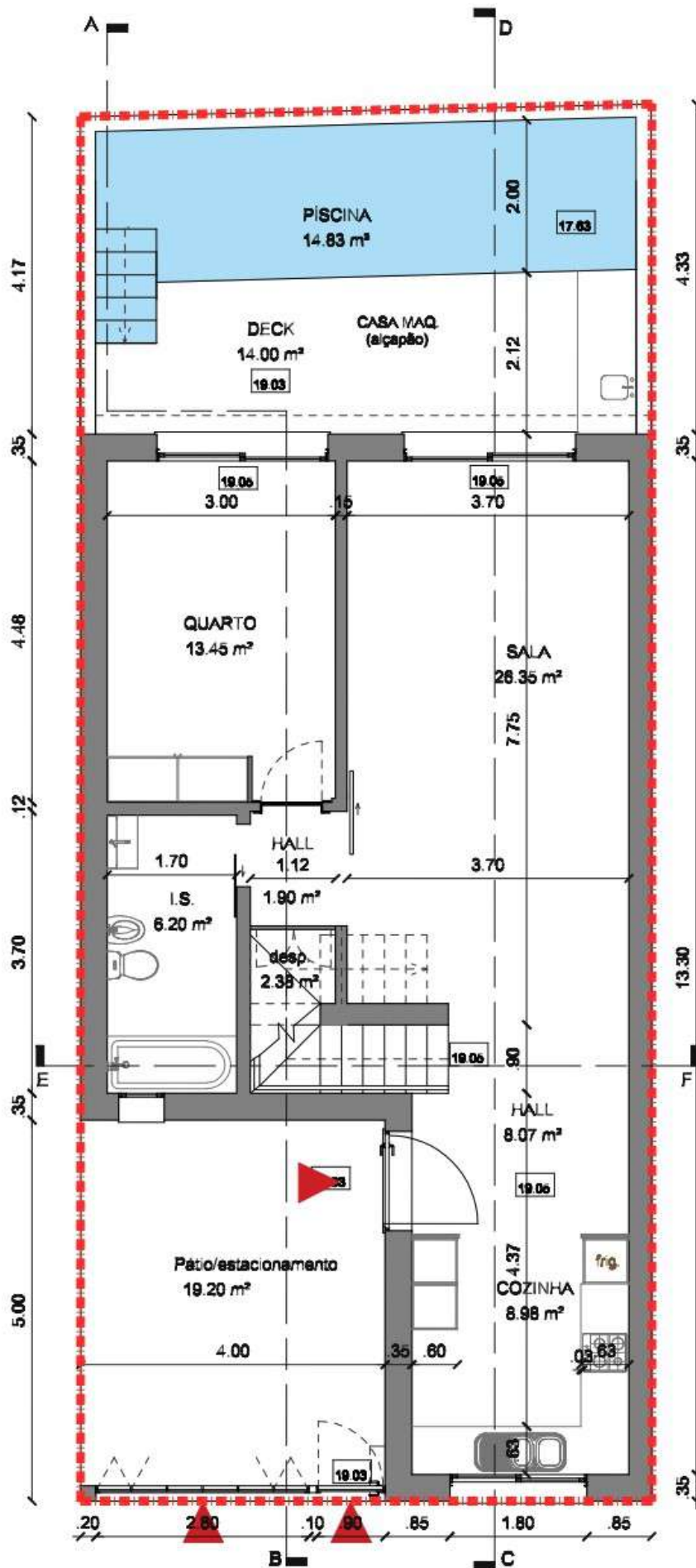
Planta Rés-do-Chão
