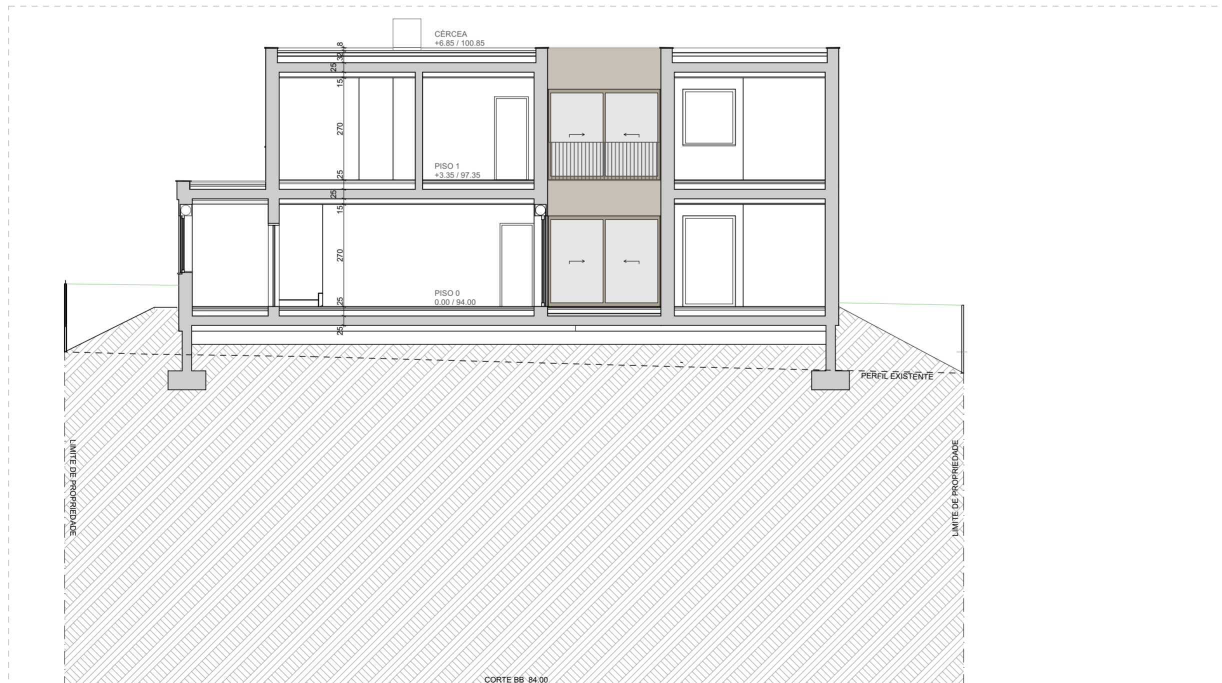
CORTE BB
