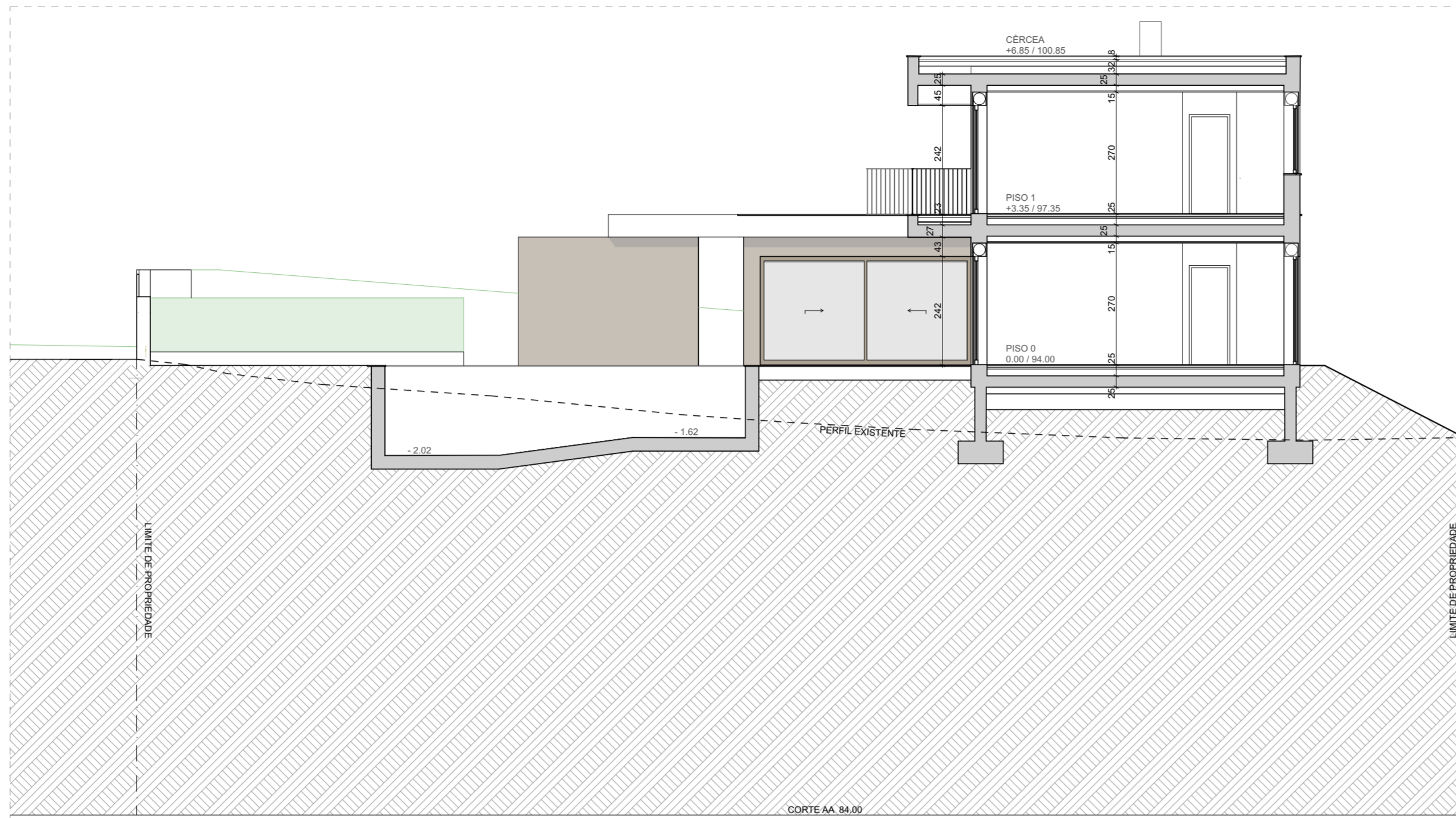
CORTE AA
