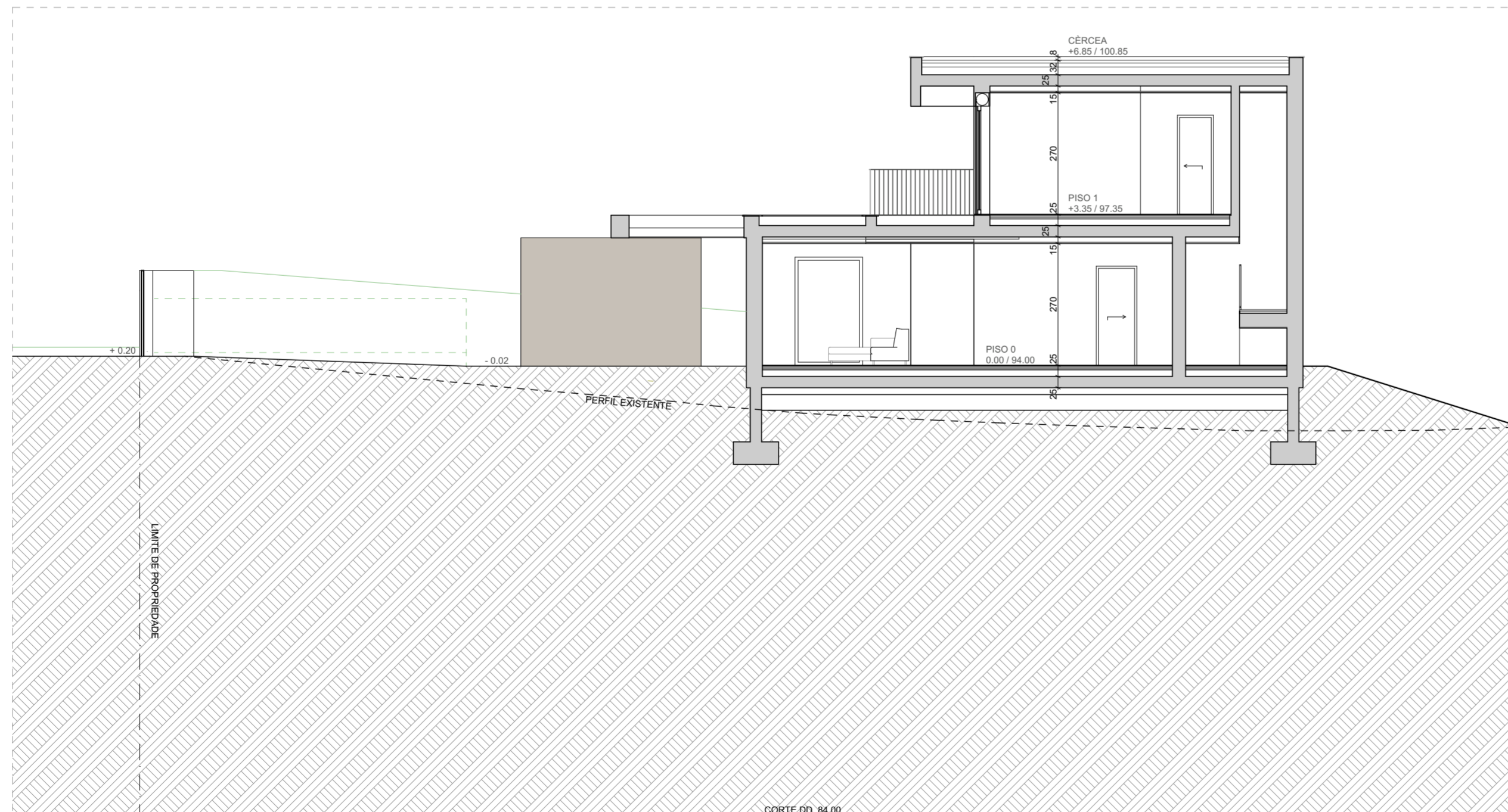
CORTE DD
