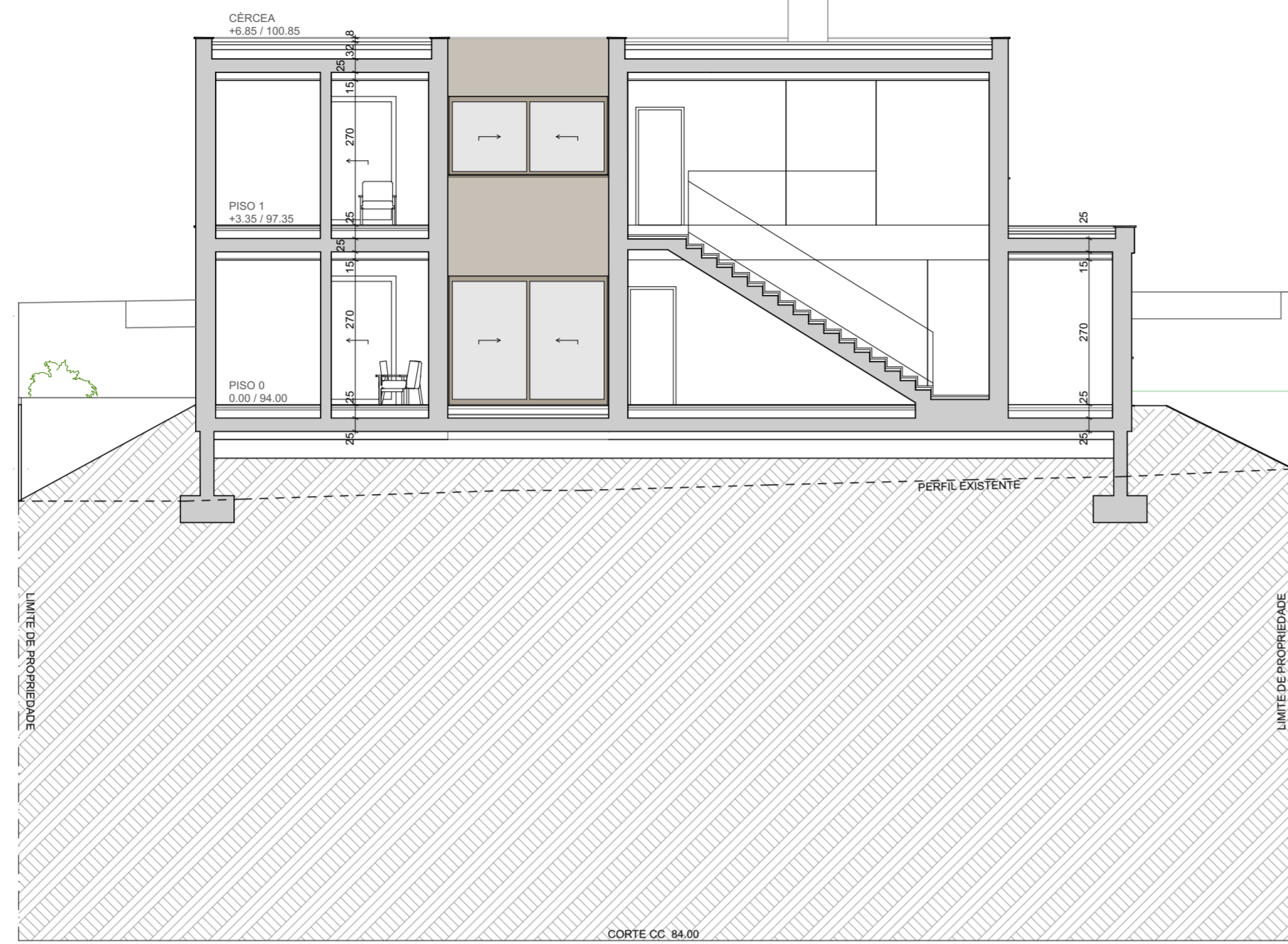
CORTE CC
