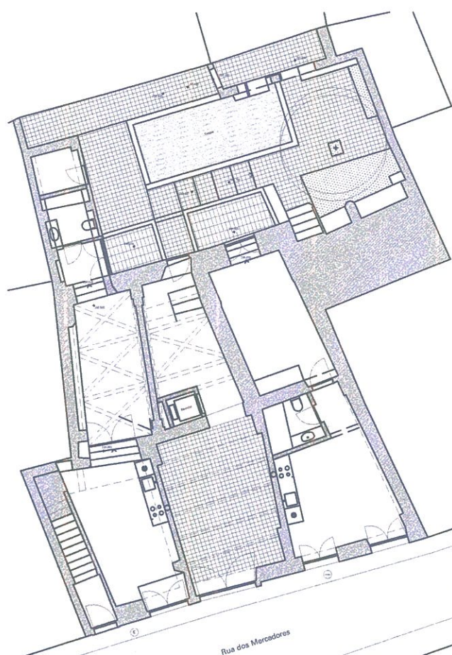
PLANTA DO PISO TÉRREO (ACESSO) ESCALA 1:200
