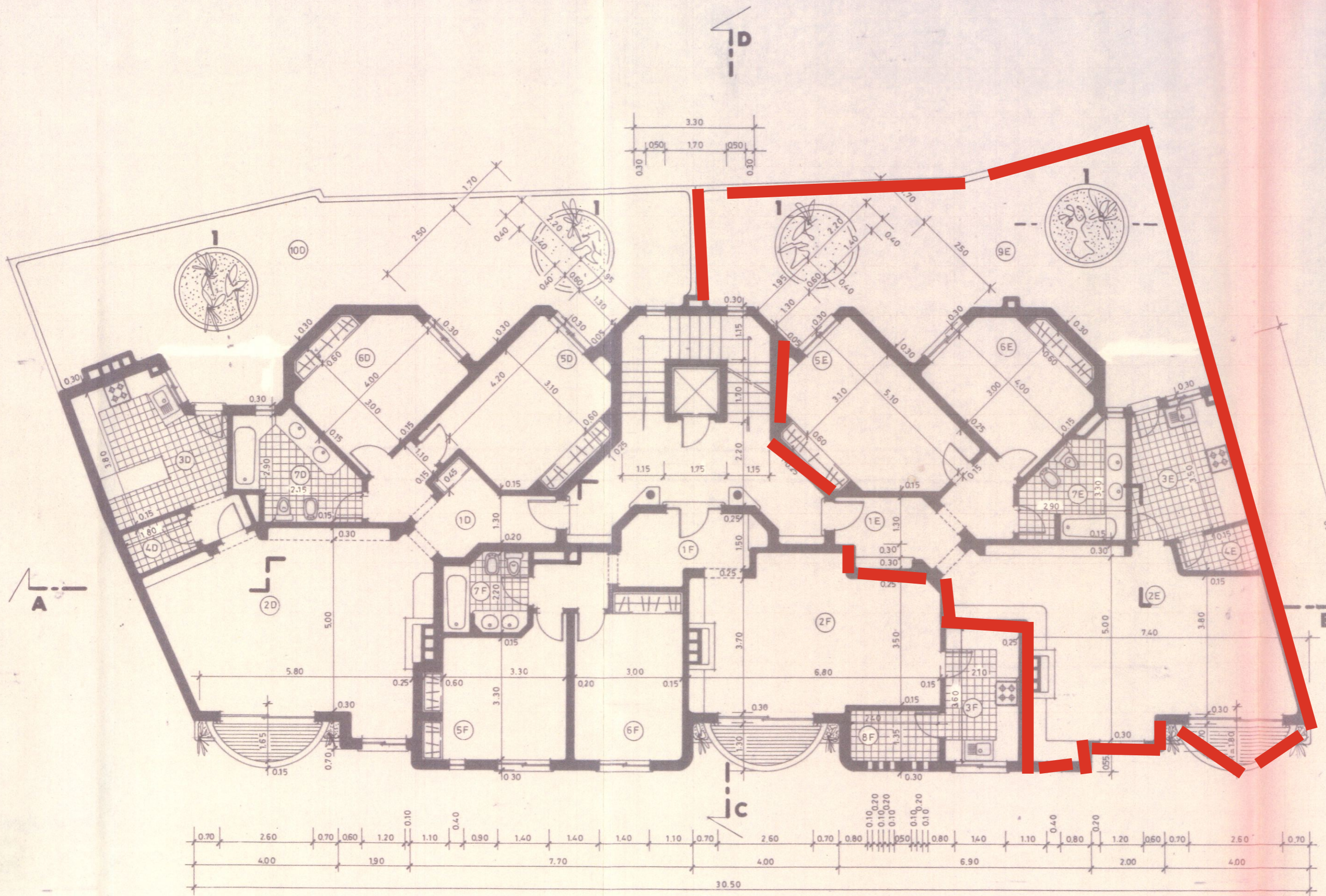
PLANTA DO 1º ANDAR
