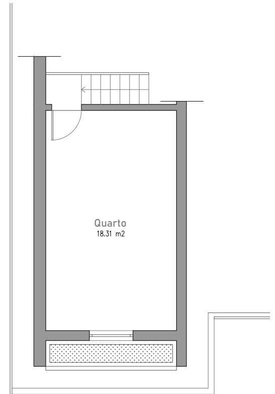
Planta do Piso 2
