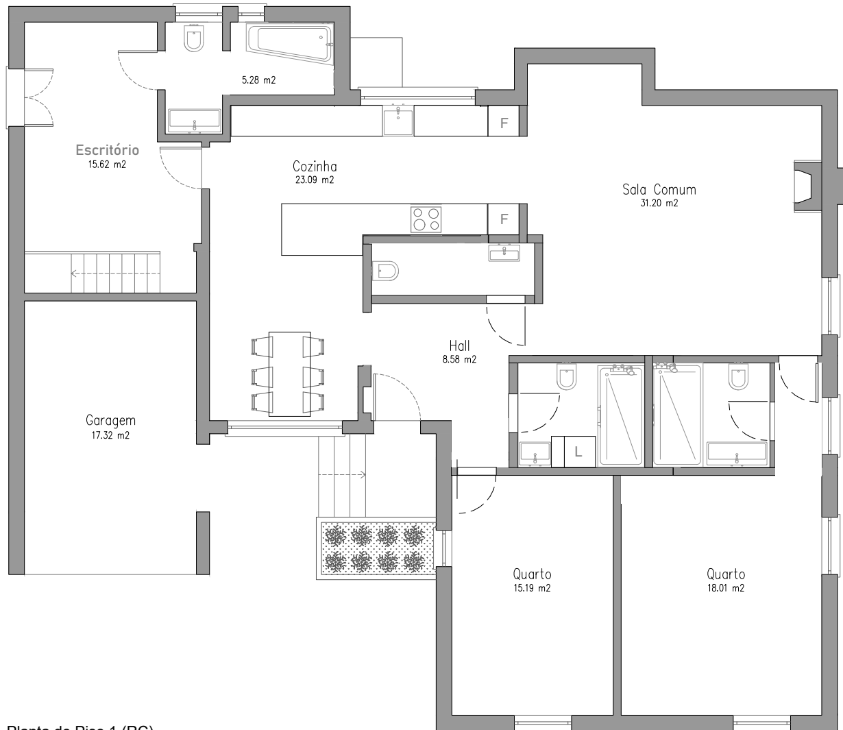
Planta do Piso 1 (RC)
